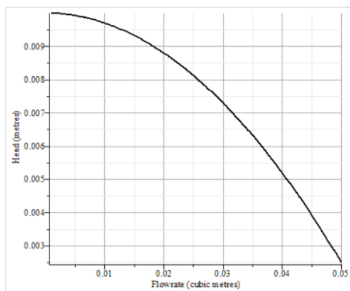
図6.32 水頭流量
