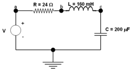
図1.5 RLC 回路
