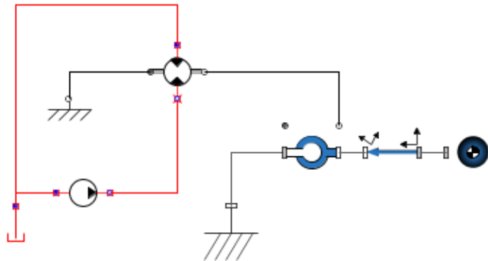
図6.22 固定回転フランジ油圧コンポーネント
