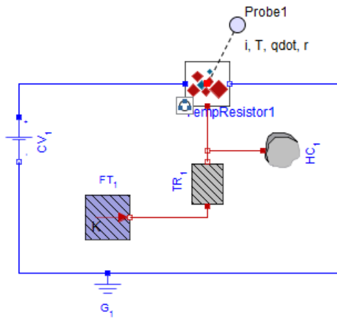
図6.4 温度依存抵抗
