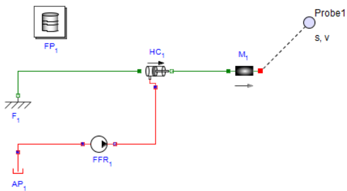
図6.18 固定流量源
